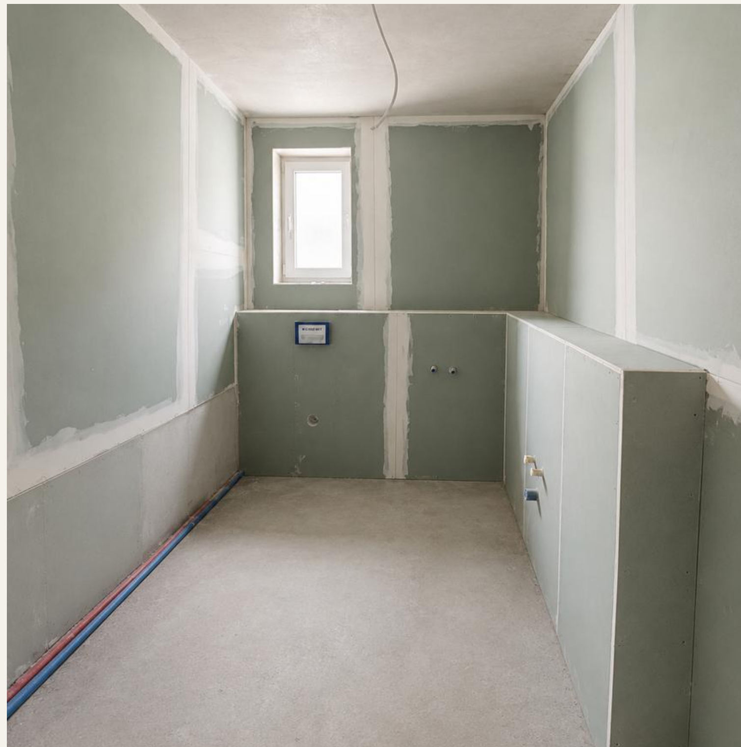
Gäste-WC & Hauswirtschaftsraum
